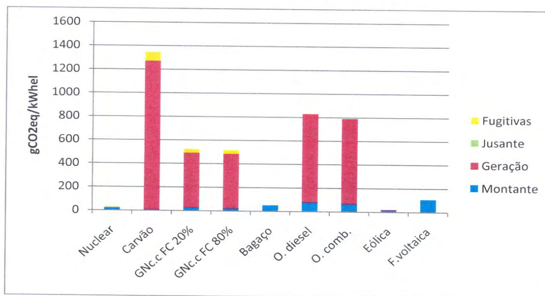
Emissões de gases do GEE por energia Elétrica gerada para o Parque brasileiro – fonte ECEN Consultoria- 2010
