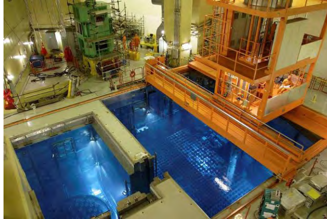
Angra 2 - Parada para troca de Combustível – 2010
